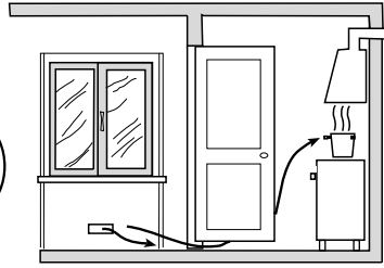
aumento de la fisura para permitir la entrada correcta del aire desde el local adyacente
