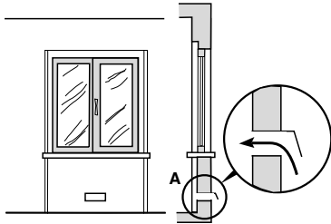
apertura de ventilación para el aire necesaria para una combustión correcta
