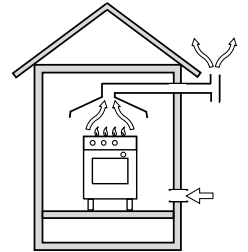
evacuación mediante chimenea reservada a la cocina
